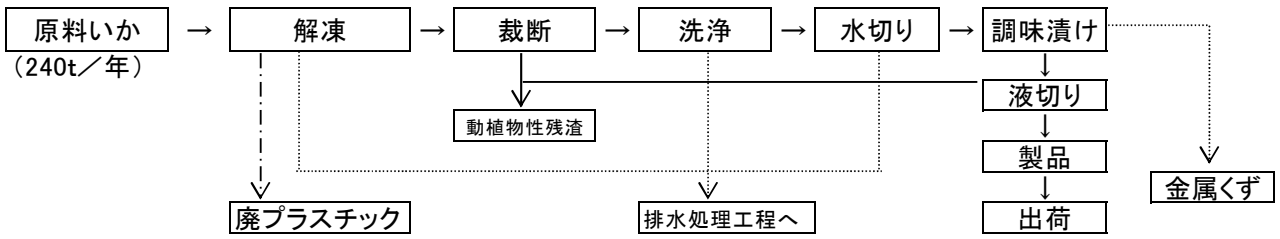
図1 いか製品製造フローシート(No.1)
