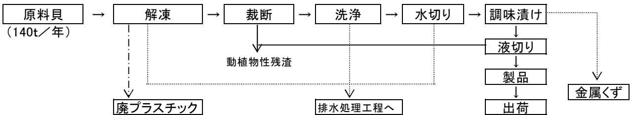
図3 貝製品製造フローシート(No.3)
